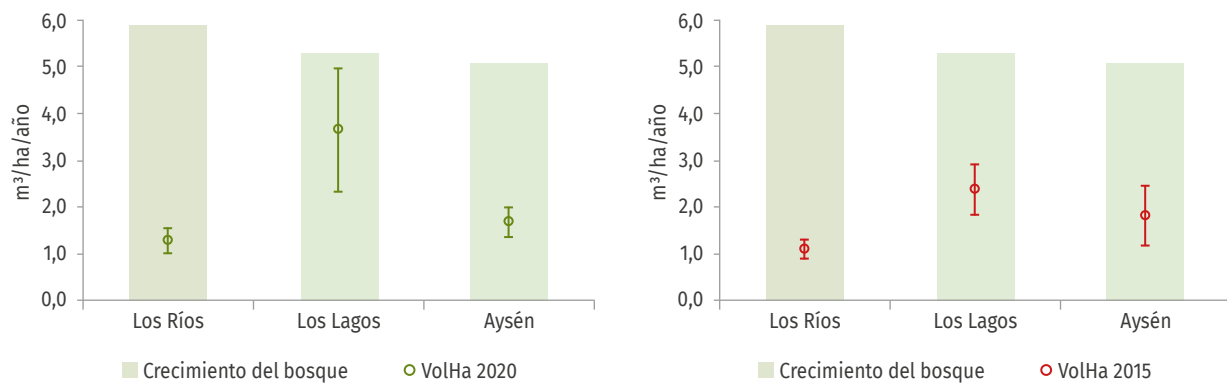
Figura 10 VOLUMEN DE MADERA NATIVA COSECHADO EN 2015 (derecha en rojo) Y 2020/23 (izquierda en verde) (tasa promedio y error estándar) Y CRECIMIENTO PROMEDIO DEL BOSQUE (columna verde)
