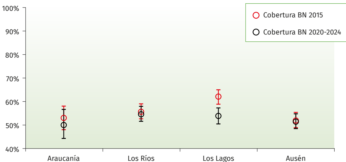
Figura 9 COBERTURA DE BOSQUE NATIVO EN LAS EXPLOTACIONES EN 2015 Y 2020/24 EN LAS REGIONES DE LA ARAUCANÍA, LOS RÍOS, LOS LAGOS Y AYSÉN (promedio y error estándar)
