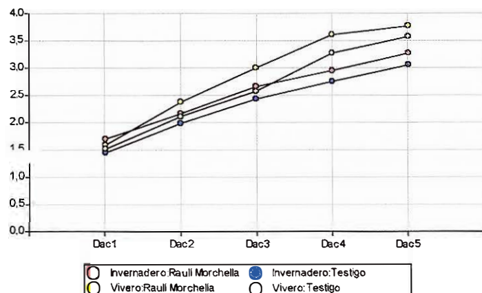
Figura 2. Perfiles temporales por tratamiento para el Dac de Raulí.
