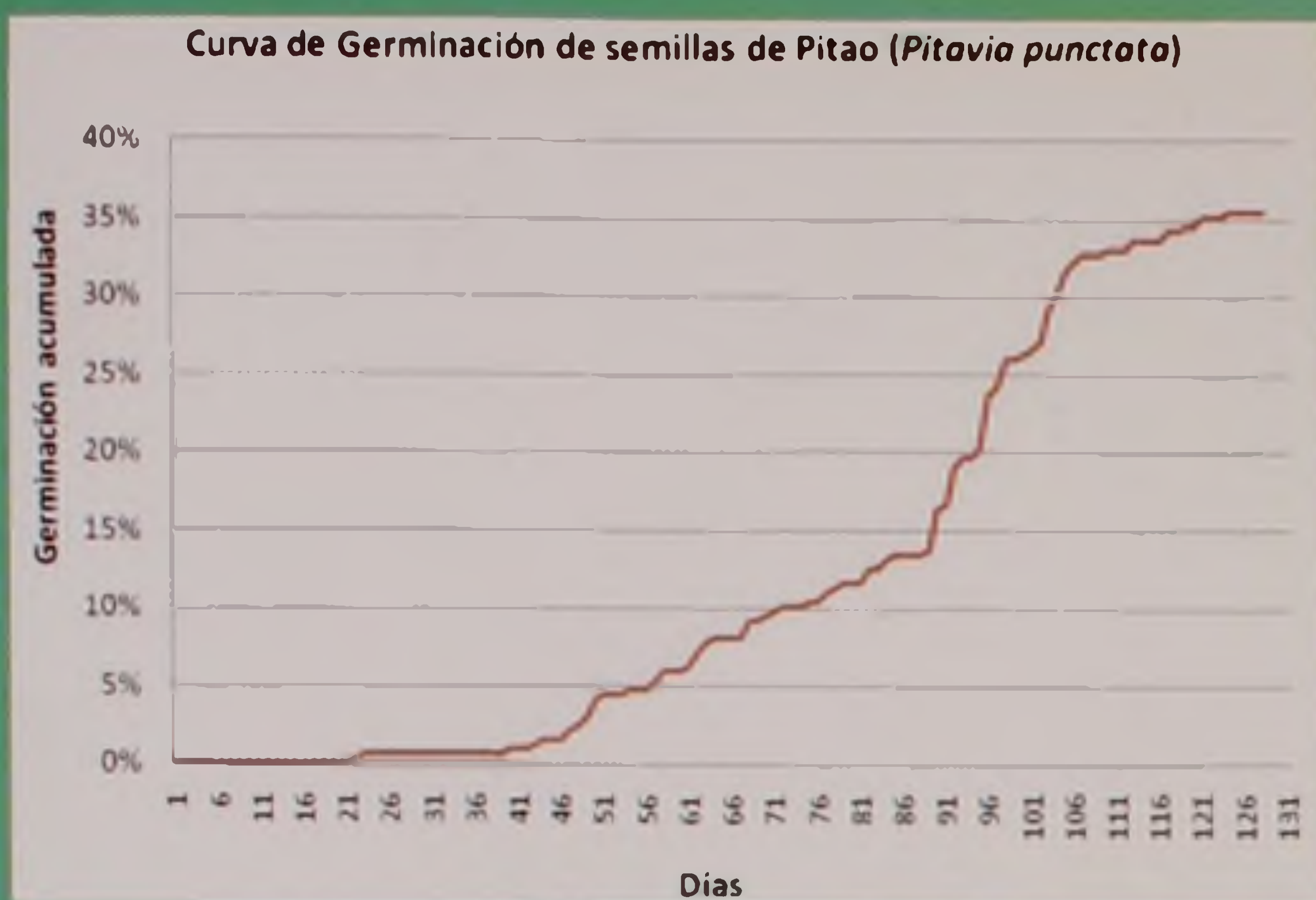
Curva de germinación acumulada de semillas de Pitavia punctata colectada en Cauquenes.
