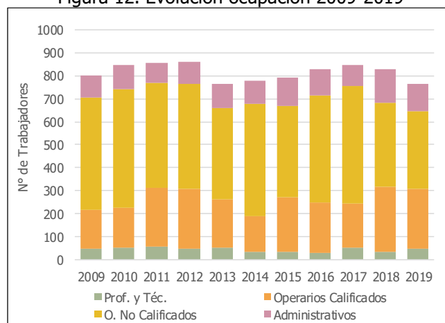
Figura 12. Evolución ocupación 2009-2019
