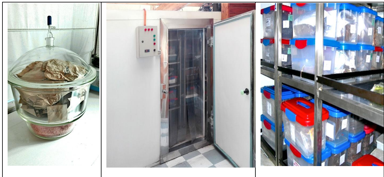
Figura 10. Desecador de sílica gel (izquierda); vista exterior e interior de cámara de frío para almacenamiento de semillas de INFOR Biobío (centro y derecha).
