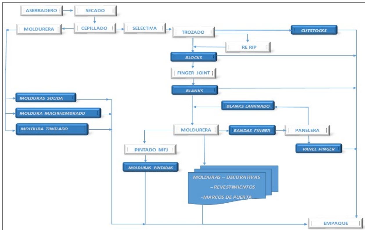
Figura 4. Lay out del proceso de fabricación de molduras de madera
