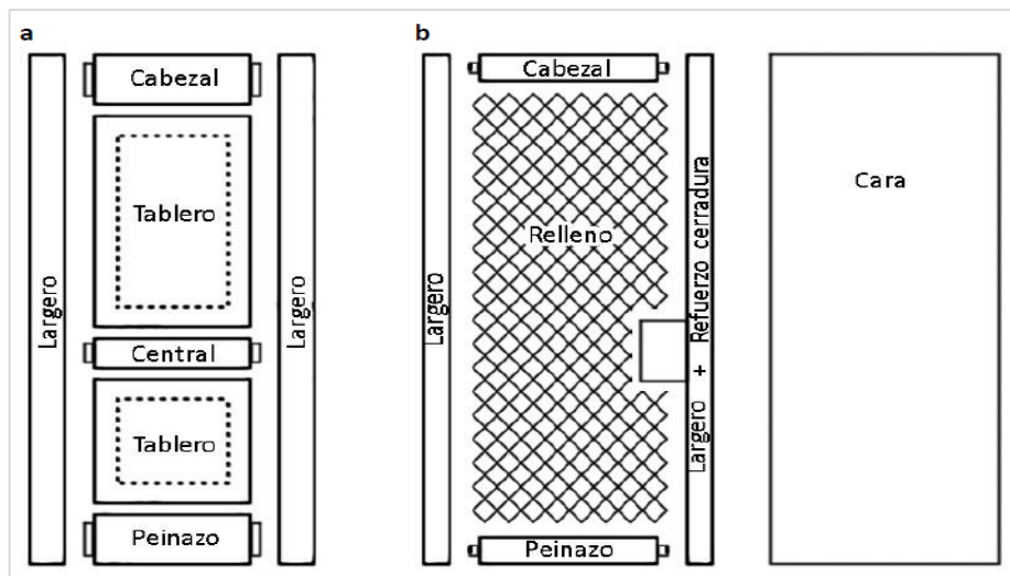
Figura 1. Composición de puerta maciza (a) y contraplacada (b)
