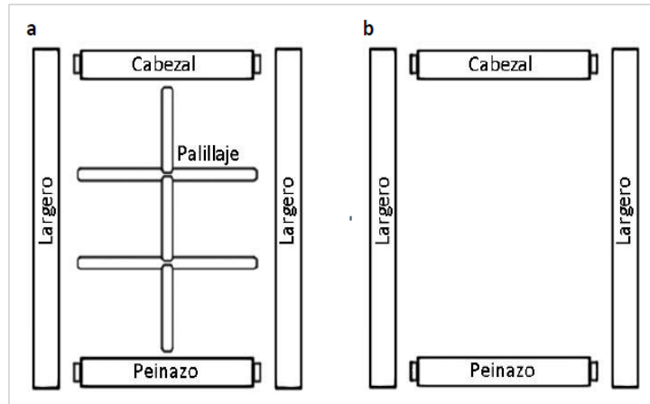
Figura 2. Composición de una ventana, con y sin palillaje
