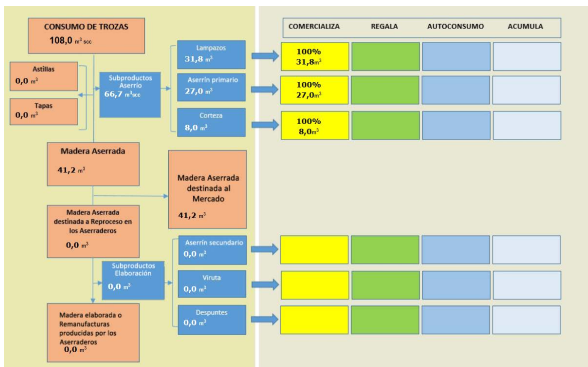
Figura 28. Región Metropolitana. Flujo de producción de madera aserrada y subproductos del aserrío, 2024
