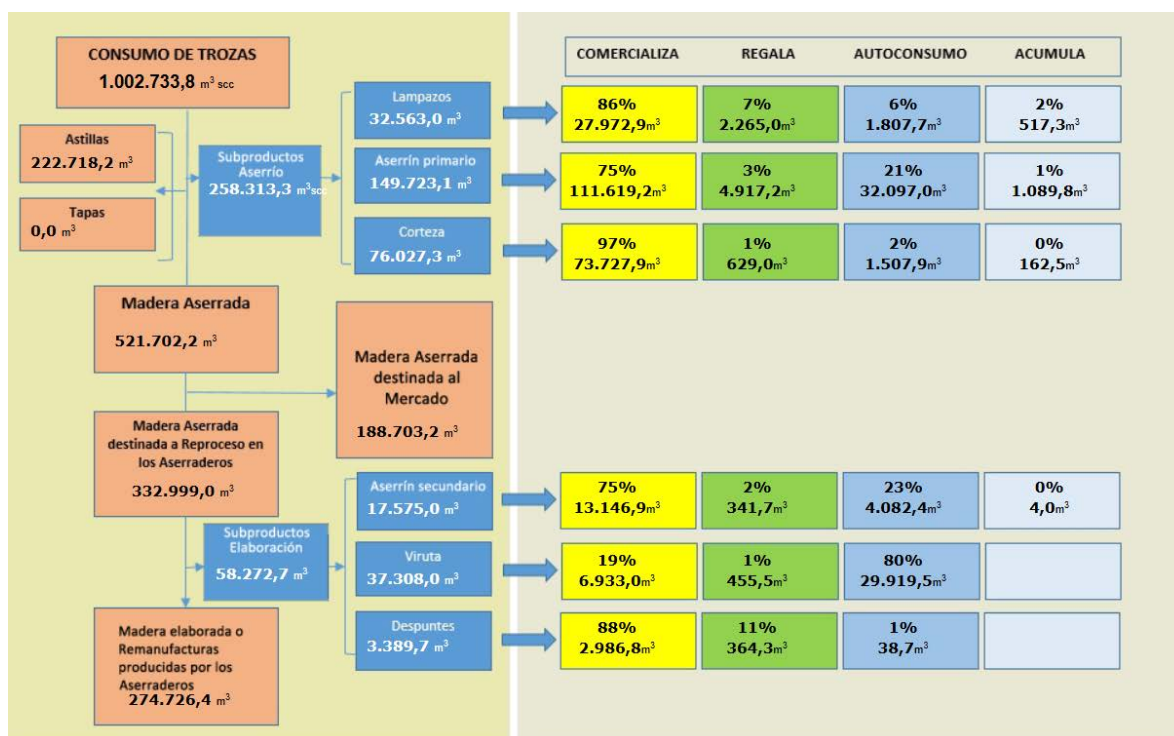
Figura 34. Región de Los Ríos. Flujo de producción de madera aserrada y subproductos del aserrío, 2024
