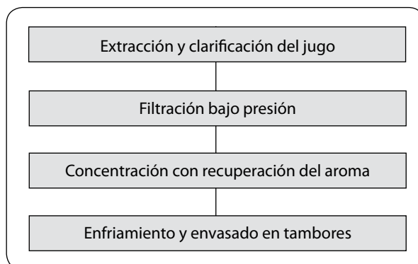
Figura 13. Diagrama de flujo del proceso de elaboración de jugos concentrados de berries (INTEC, 1986; Valdebenito et al., 2006).
