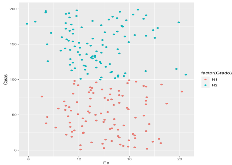
Figura A17 DISPERSIÓN DE DATOS MÓDULO DE ELASTICIDAD FLEXIÓN (MPa)
