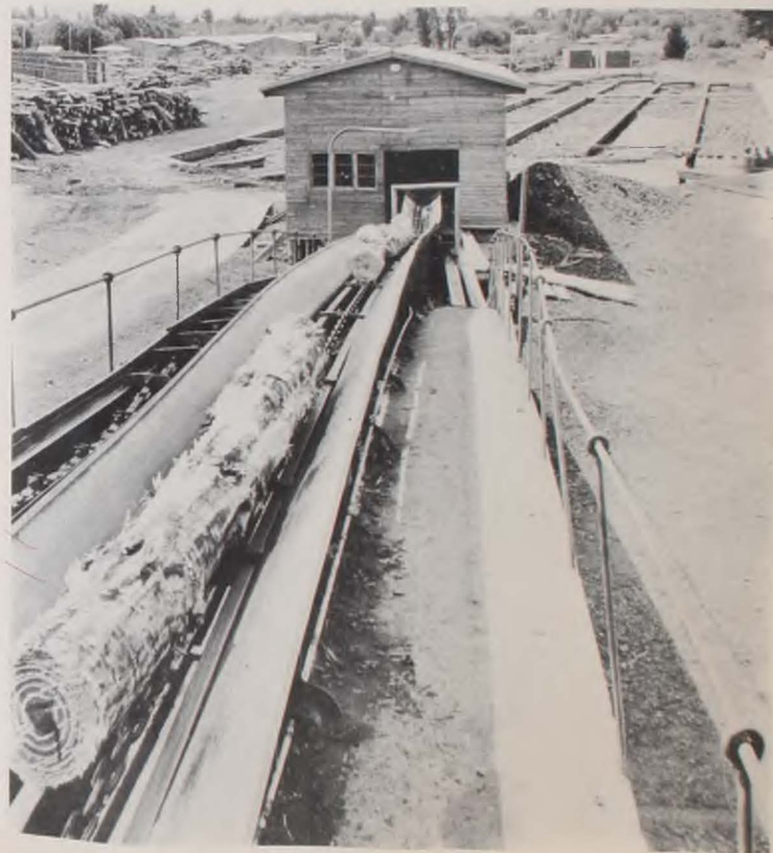
Cadena transportadora de trozas alimentando un aserradero alternativo
