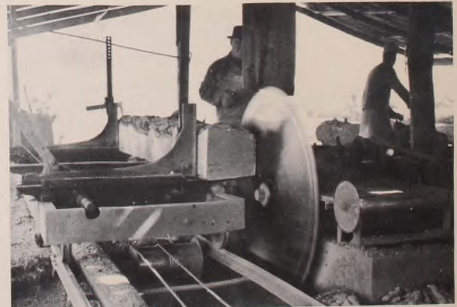
Aserradero de sierra circular para pino insigne, de tipo portátil
