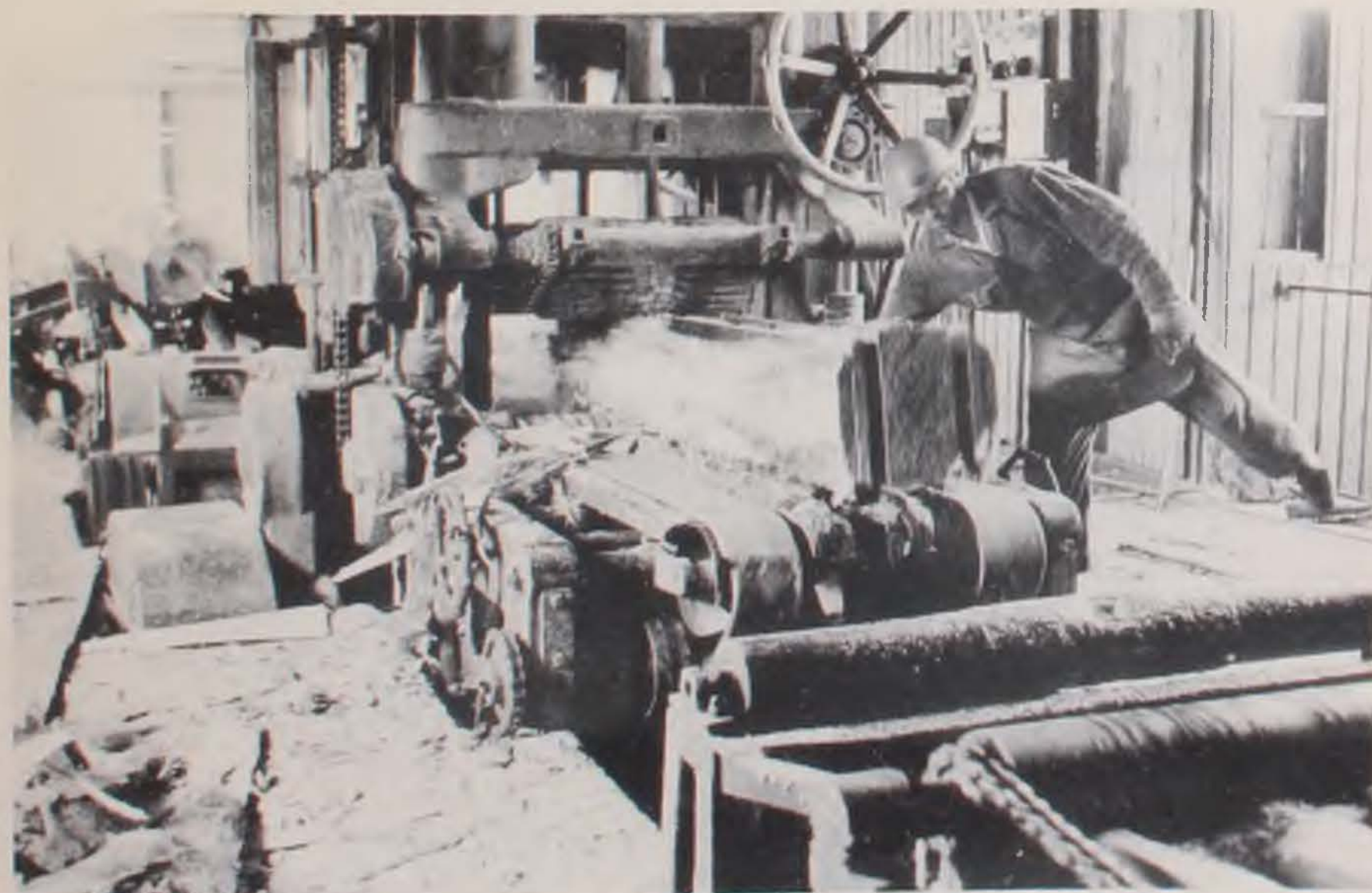
Aserradero alternativo empleado en plantaciones.
