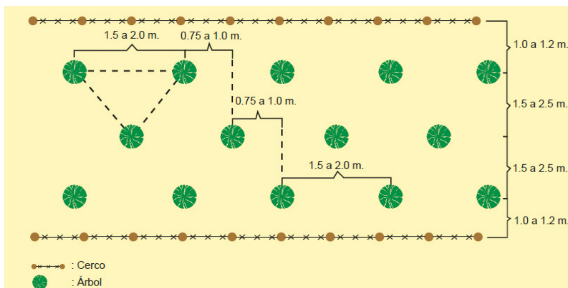
Figura N° 48 EJEMPLO DE MARCO DE PLANTACIÓN DE CORTINA CORTAVIENTO CON DISTANCIAMIENTOS PARA ESTABLECER UNA CORTINA DE TRES HILERAS CON PLANTACIÓN EN TRES BOLILLO
