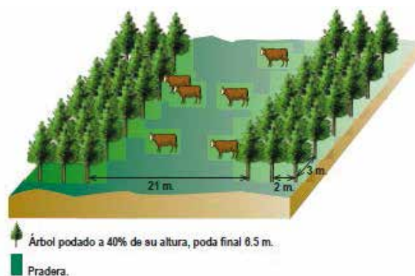
Figura N° 10 ESTABLECIMIENTO EN ARREGLO SILVOPASTORAL EN FAJAS
