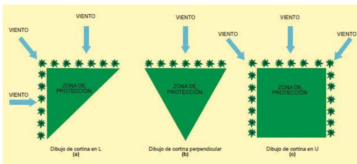
Figura N° 49 DISEÑO Y ORIENTACIÓN DE CORTINAS SEGÚN DIRECCIÓN DEL VIENTO.
