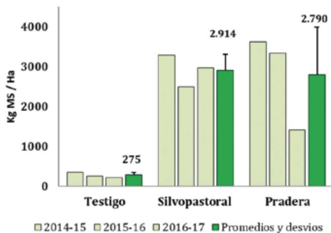
Figura N° 40 PRODUCCIÓN DE LA PRADERA EN TRATAMIENTO TESTIGO; EN MANEJO SILVOPASTORAL DE ÑIRRE, Y EN PRADERA SIN ÁRBOLES
