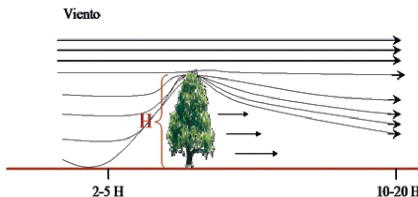
FIGURA N° 47 MOVIMIENTO DEL AIRE A TRAVÉS DE LA CORTINA Y SOBRE ESTA
