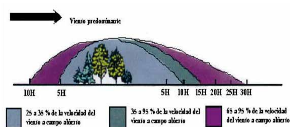
Figura N° 43 PORCENTAJE DE REDUCCIÓN DE VELOCIDAD DEL VIENTO EN UNA CORTINA CORTAVIENTO CUYA ALTURA ES H
