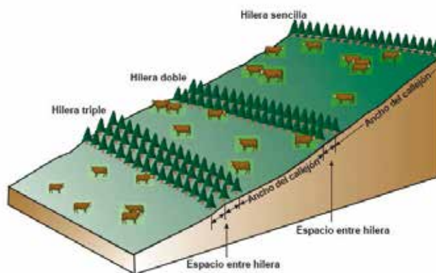
Figura N° 6 CONFIGURACIÓN DE PLANTACIÓN DE HILERAS SIMPLES, DOBLES Y TRIPLES PARA UN SISTEMA SILVOPASTORAL
