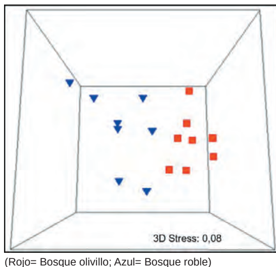
Figura N° 1 DIAGRAMA DE SIMILITUD FLORÍSTICA DE LAS FORMACIONES VEGETACIONALES IDENTIFICADAS EN PREDIO PUMILLAHUE
