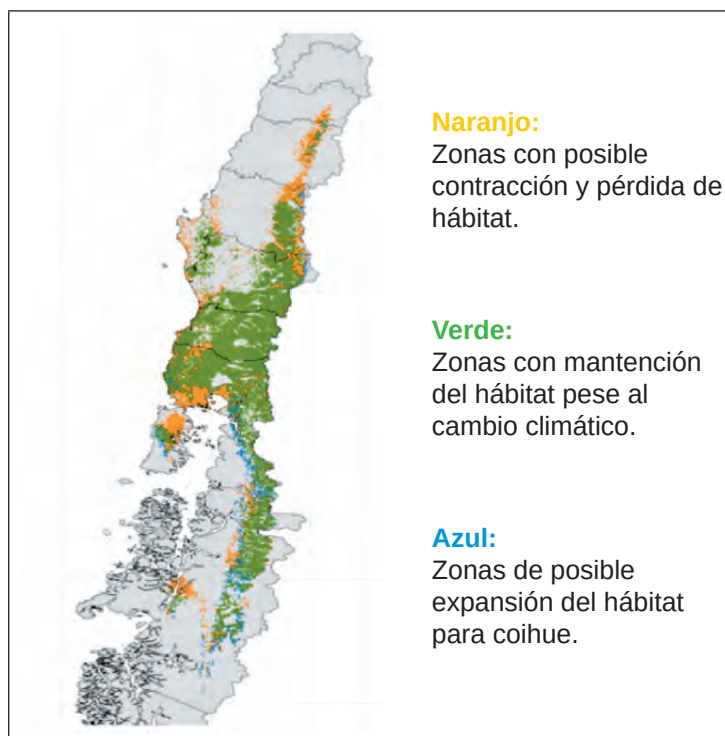
Figura N° 4 ESQUEMA DE LA DISTRIBUCIÓN DEL HÁBITAT DE COIHUE SEGÚN VULNERABILIDAD AL CAMBIO CLIMÁTICO
