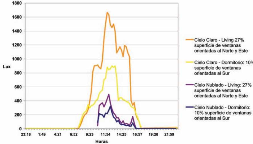
GRÁFICO 7. Iluminación Natural al Interior de los Recintos Según Tipo de Cielo y Orientación en el Valle Central
