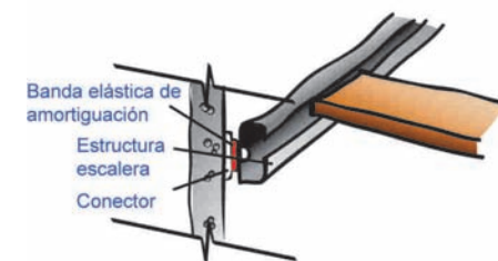
Control de la transmisión de ruido a través del adosamiento de la escalera al muro medianero
