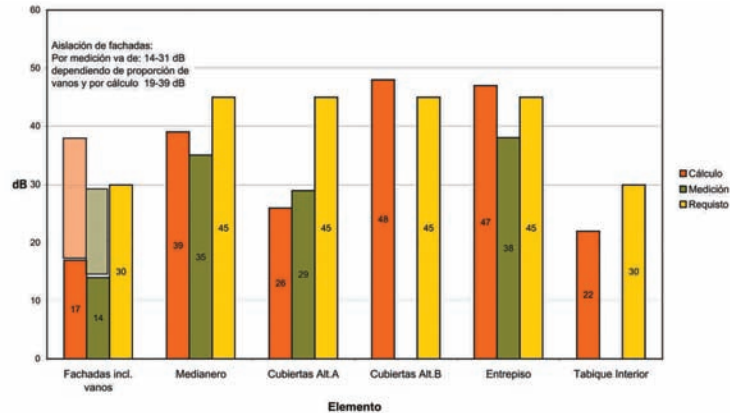
GRÁFICO 6. Aislación Acústica al Ruido Aéreo dB
