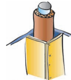
Encajonamiento de descarga con tubo embarrilado en fibra
