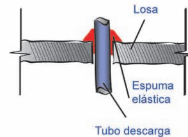
Amortiguador
