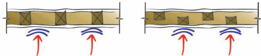
Pies derechos desfasados pueden aumentar la aislación acústica en aproximadamente 5 dB
