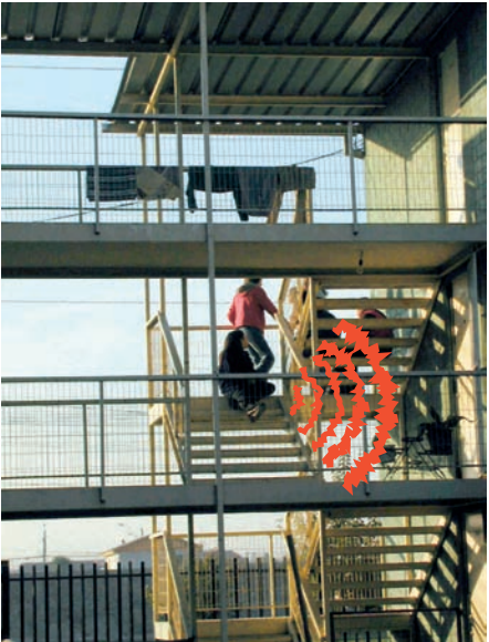
Ruido por empotramiento estructural de la escalera
