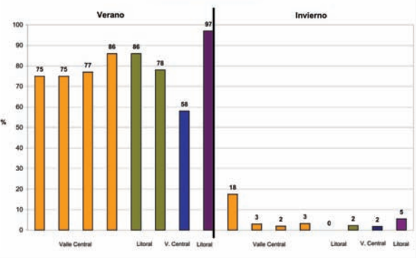
GRÁFICO 2. Habitabilidad Térmica. Viviendas deshabitadas
