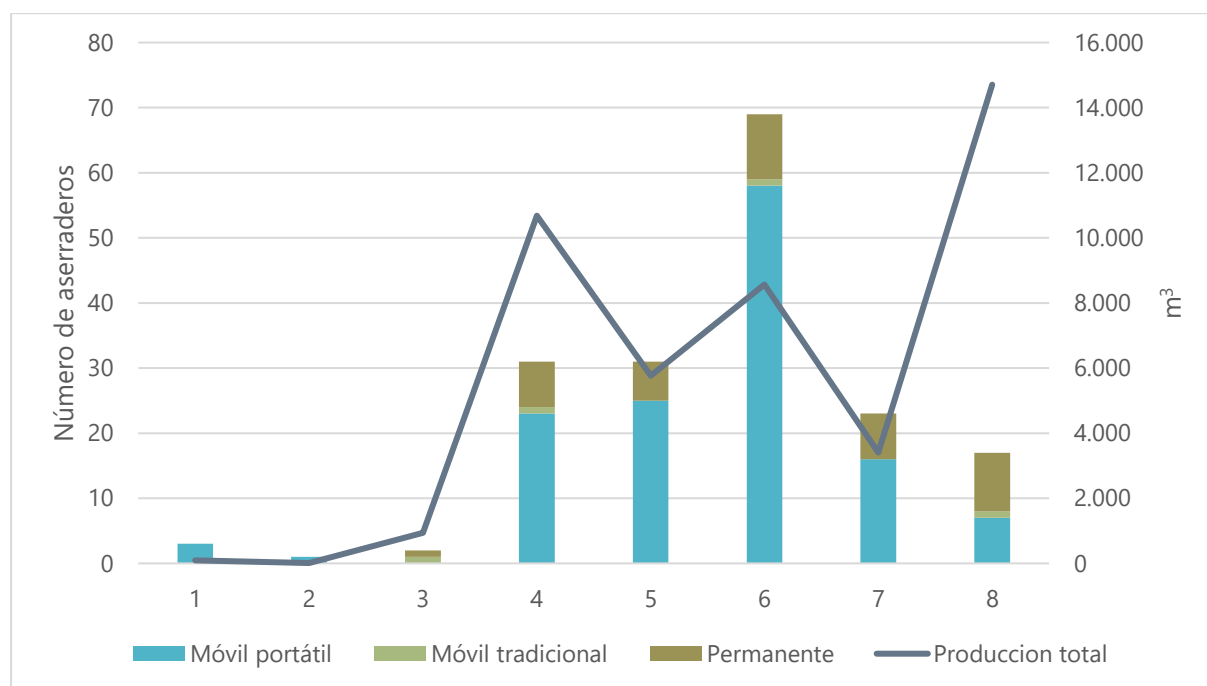
Figura 2. Número de aserraderos que procesan especies nativas por tipo de aserradero, según región y producción anual, 2024.
