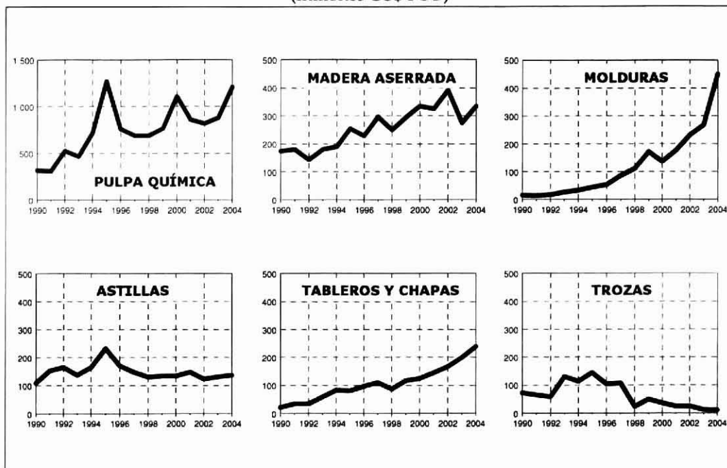
Figura 4.6 EVOLUCIÓN DE LAS EXPORTACIONES FORESTALES, SEGÚN PRODUCTO (millones US$ FOB)
