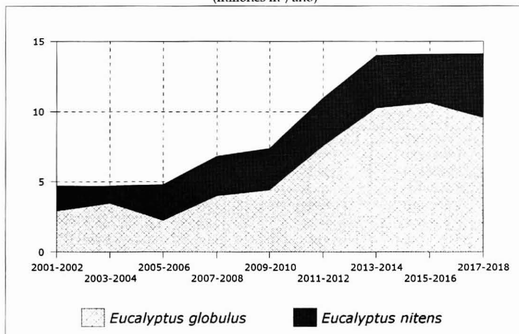
Figura 7.2 DISPONIBILIDAD DE EUCALIPTO TOTAL Y POR ESPECIE (millones m 3 /año)
