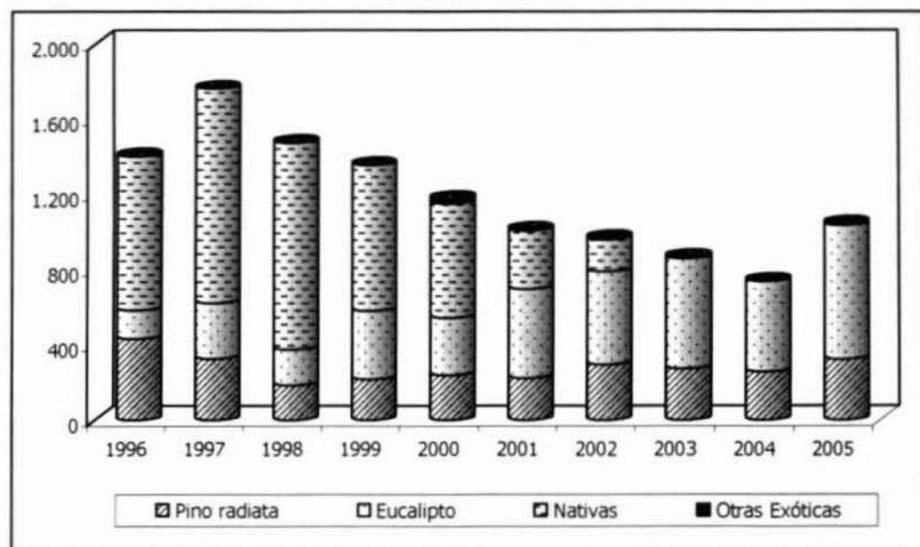
Figura 3.2 EVOLUCIÓN DE LA PRODUCCIÓN DE ASTILLAS (miles m 3 ssc)
