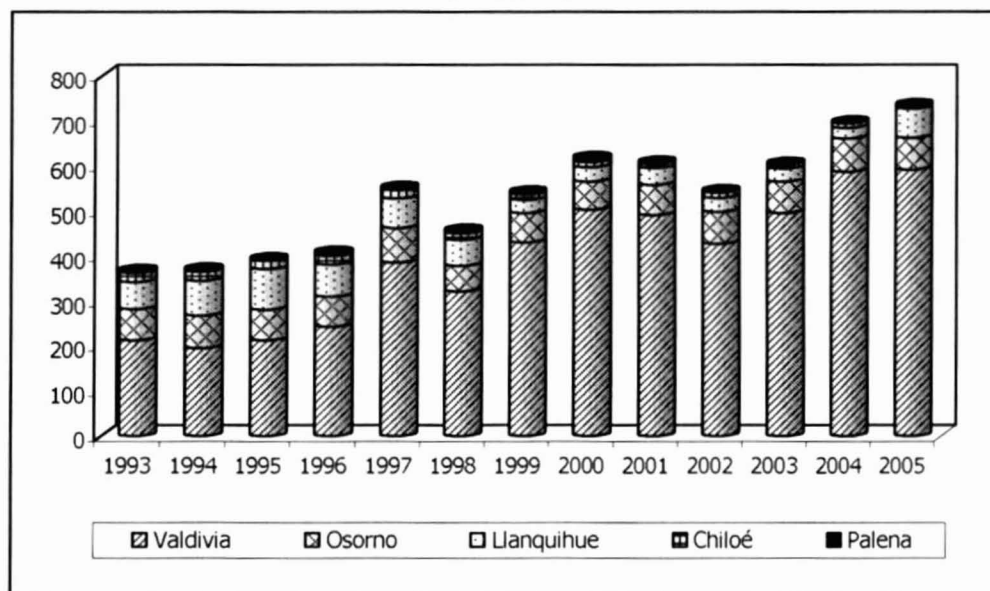
Figura 3.1 PRODUCCIÓN DE MADERA ASERRADA POR PROVINCIA (miles m 3 )
