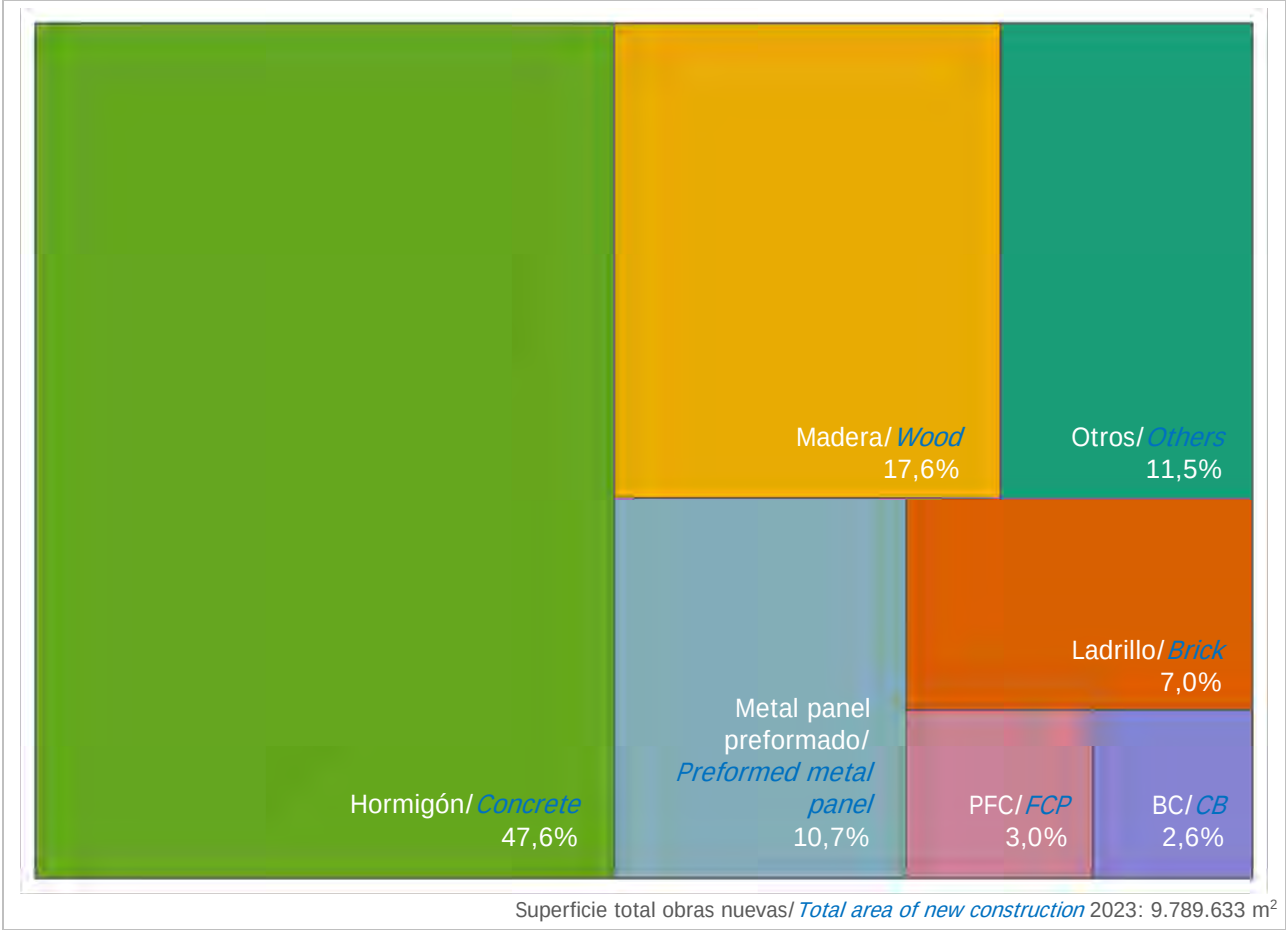
Figura 1.3. Participación de los materiales predominante en muros, en la superficie autorizada habitacional y no habitacional de obras nuevas, 2023.
