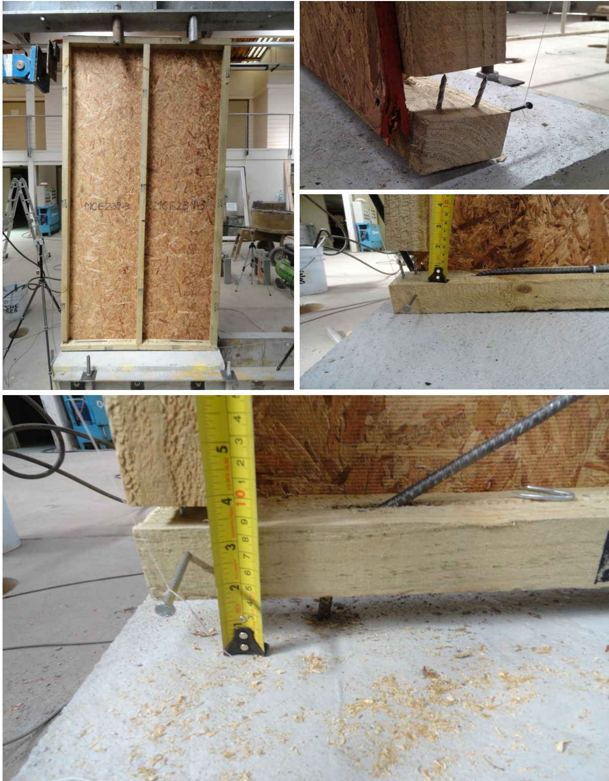
Figura 2.17: Modo de falla característico de ensayo de carga horizontal en muros con estructura de madera con sistema de anclaje espárrago
