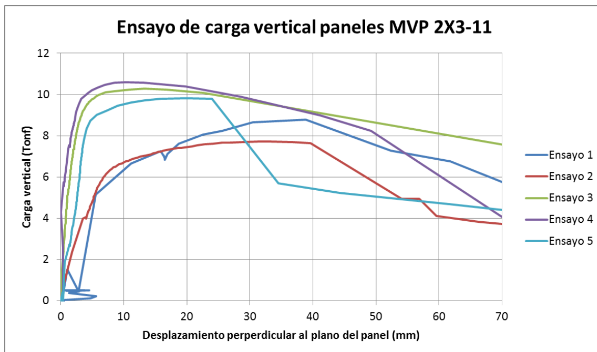
Figura 2.8: Gráfico carga-desplazamiento de ensayos de carga vertical en muros de tipología MP 2x3-11.
