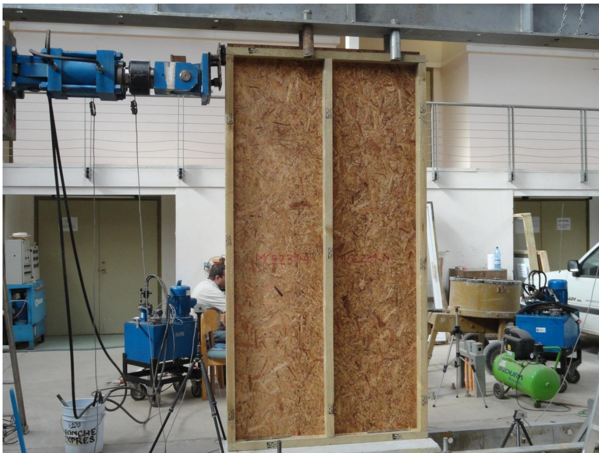
Figura 2.3: Implementación del ensayo de carga horizontal en muros con estructura de madera.
