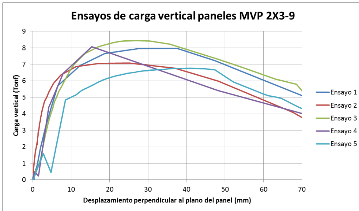
Figura 2.7: Gráfico carga-desplazamiento de ensayos de carga vertical en muros de tipología MP 2x3-9.
