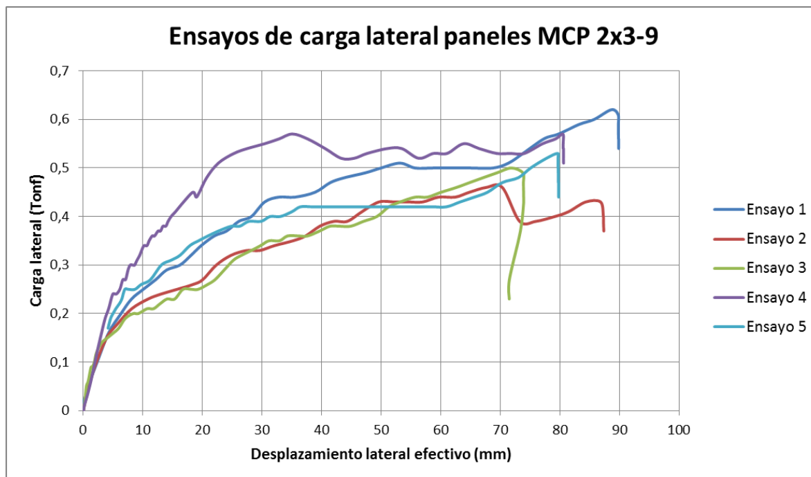
Figura 2.13: Gráfico carga-desplazamiento de ensayos de carga horizontal en muros de tipología MP 2x3-9.
