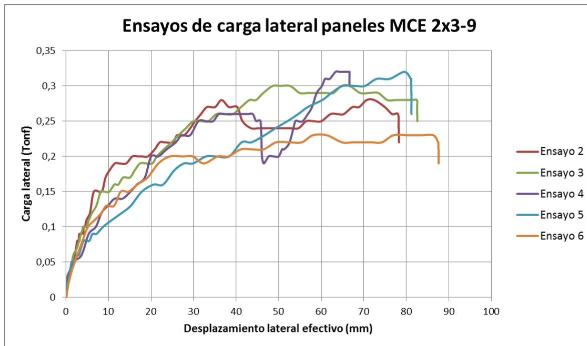
Figura 2.12: Gráfico carga-desplazamiento de ensayos de carga horizontal en muros de tipología ME 2x3-9.
